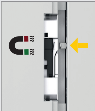
Magnet aktiviert Riegelbolzen | magnet activates locking bolt
